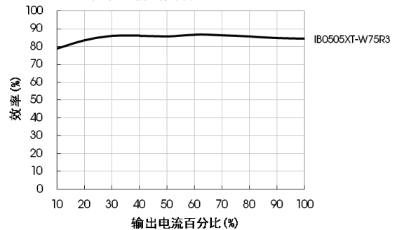
效率Vs输出负载 (Vin=5V)
